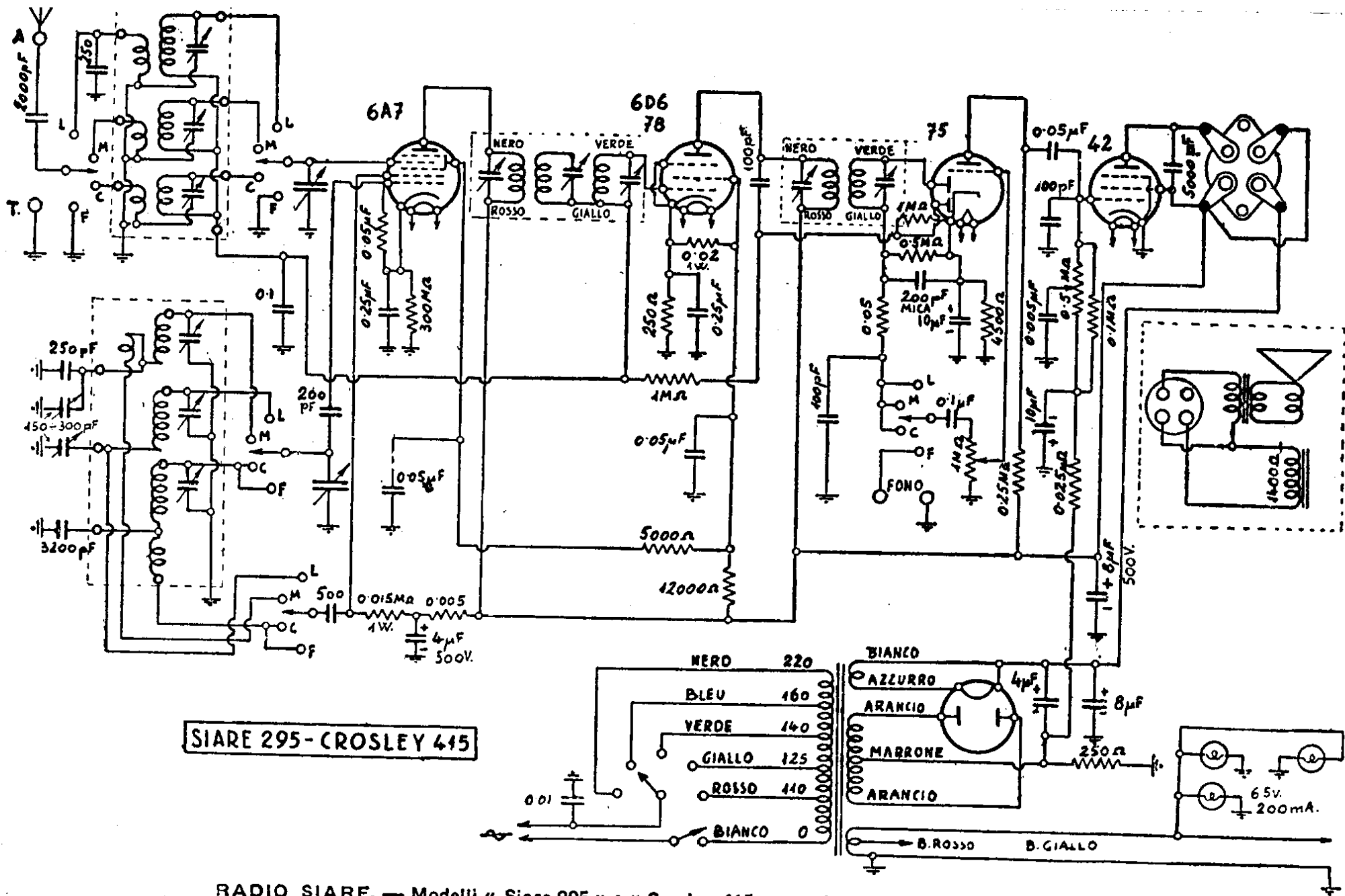
RADIO SIARE. — Modelli « Siare 295 » e « Crosley 415 » a onde corte medie e lunghe (serie panfonica). Produzione 1937. — Media frequenza: 468 kHz.
